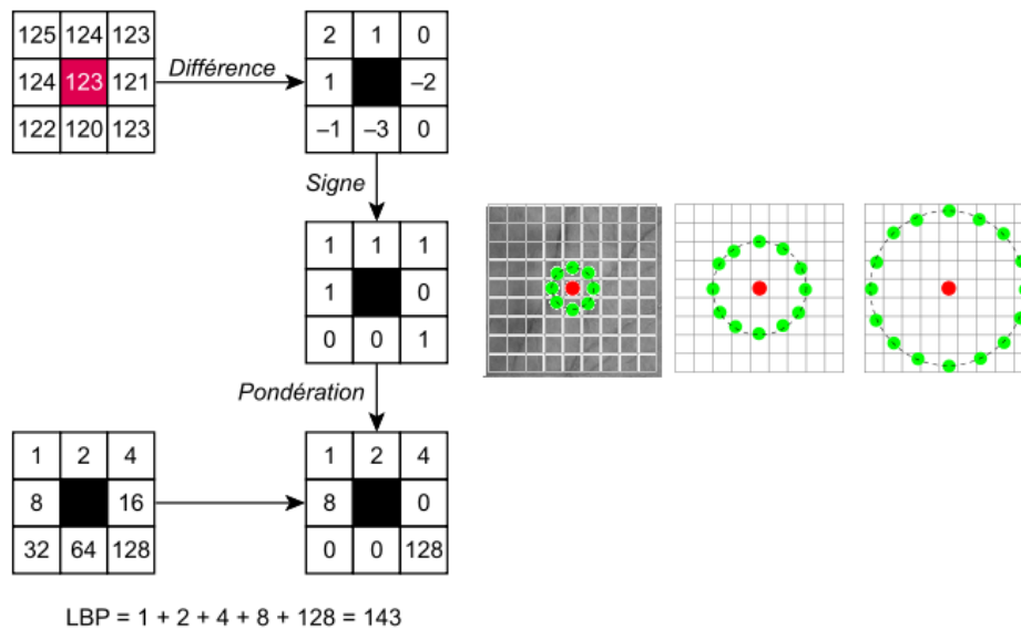
Fig 3.7 – Algorithme pour calculer un motif binaire local ou Local binary Patterns (LBP).
