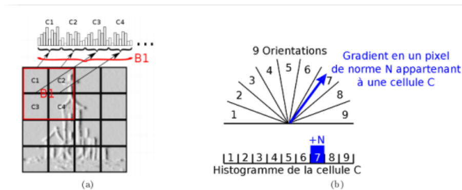
Fig 3.14 – Formation du HoG d'une image : (a) découpage en cellules et formation de l'histogramme par blocs, (b) vote d'un pixel selon l'orientation de ses gradients.
