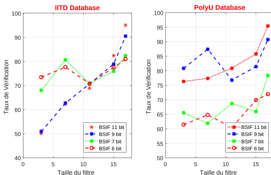
Fig 4.1 – Les taux de vérification (BSIF) en (%)
