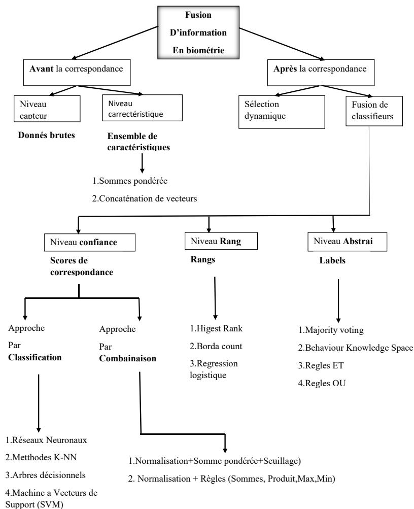
Fig 1.4 – Résumé des approches de fusion dans les systèmes biométriques multimodaux [Sanderson and Paliwal, 2002]
