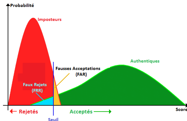
Fig 1.5 – Illustration du FRR et du FAR [Perronnin and Dugelay, 2002]
