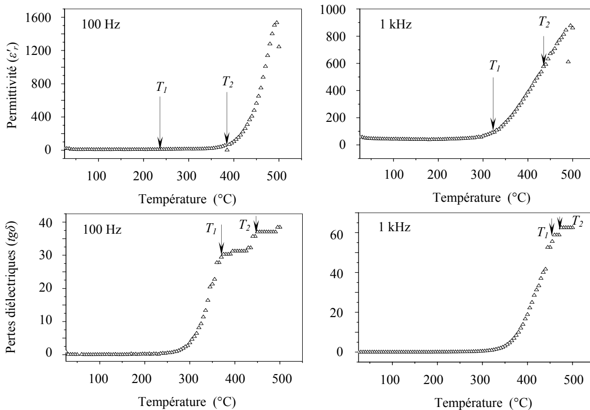
Figure 26: Variations de \epsilon'_r et tg\delta avec la température pour l'oxyfluorure
