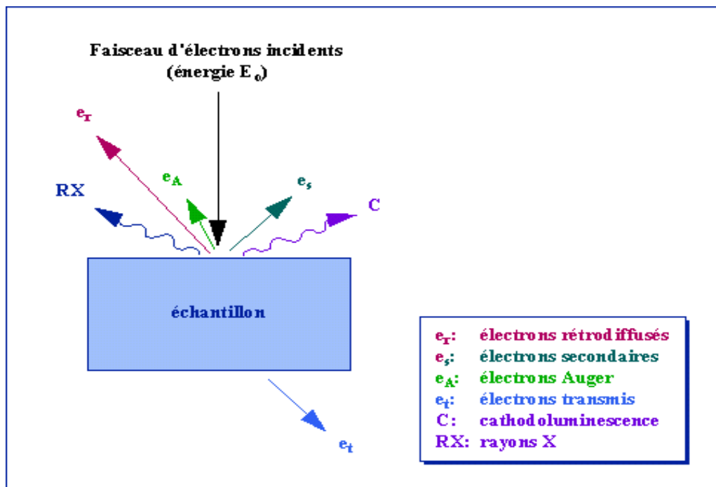
Figure 14: Représentation schématique de l'interaction entre le faisceau d'électrons et la surface de l'échantillon
