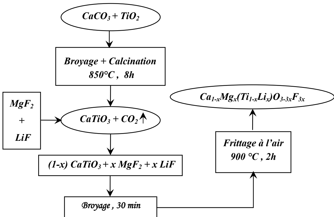
Figure 13: Protocole de préparation de CaTiO_3 et d'élaboration des céramiques Ca_{1-x}Mg_x(Ti_{1-x}Li_x)O_{3-3x}F_{3x}
