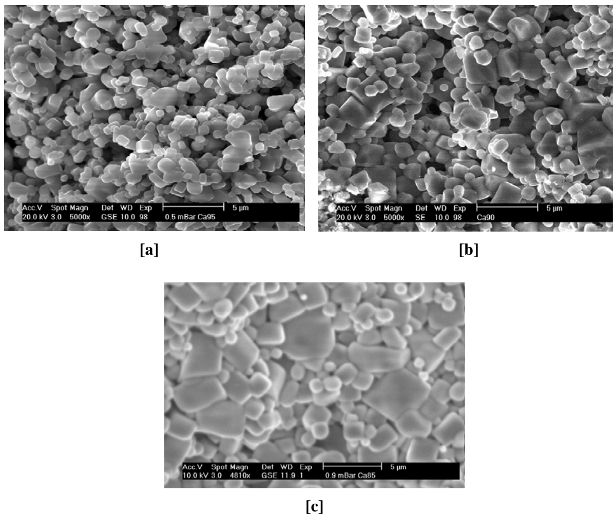
Figure 22: Microstructures des céramiques Ca_{1-x}Mg_x(Ti_{1-x}Li_x)O_{3-3x}F_{3x} frittées à 900 °C pendant 2h ([a] x = 0,05 ; [b] x = 0,10 ; [c] x = 0,15 )
