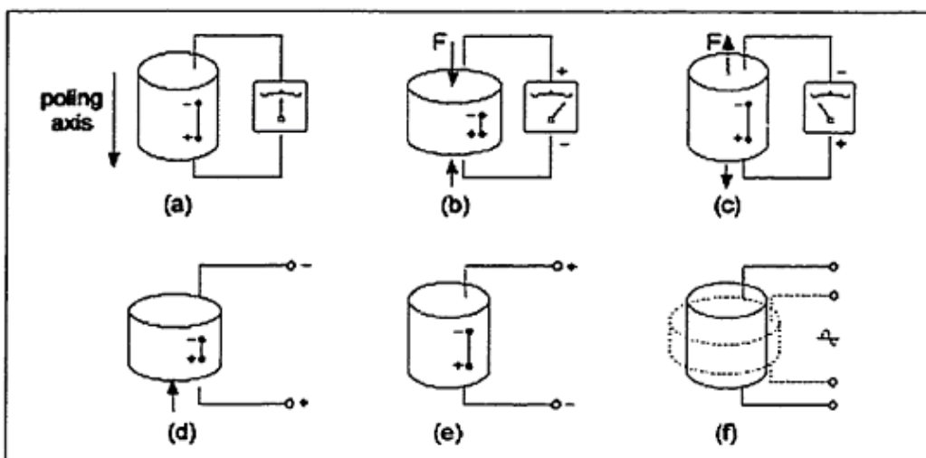
Figure 9: Effet piézoélectrique direct et inverse dans un cylindre à base de PZT
