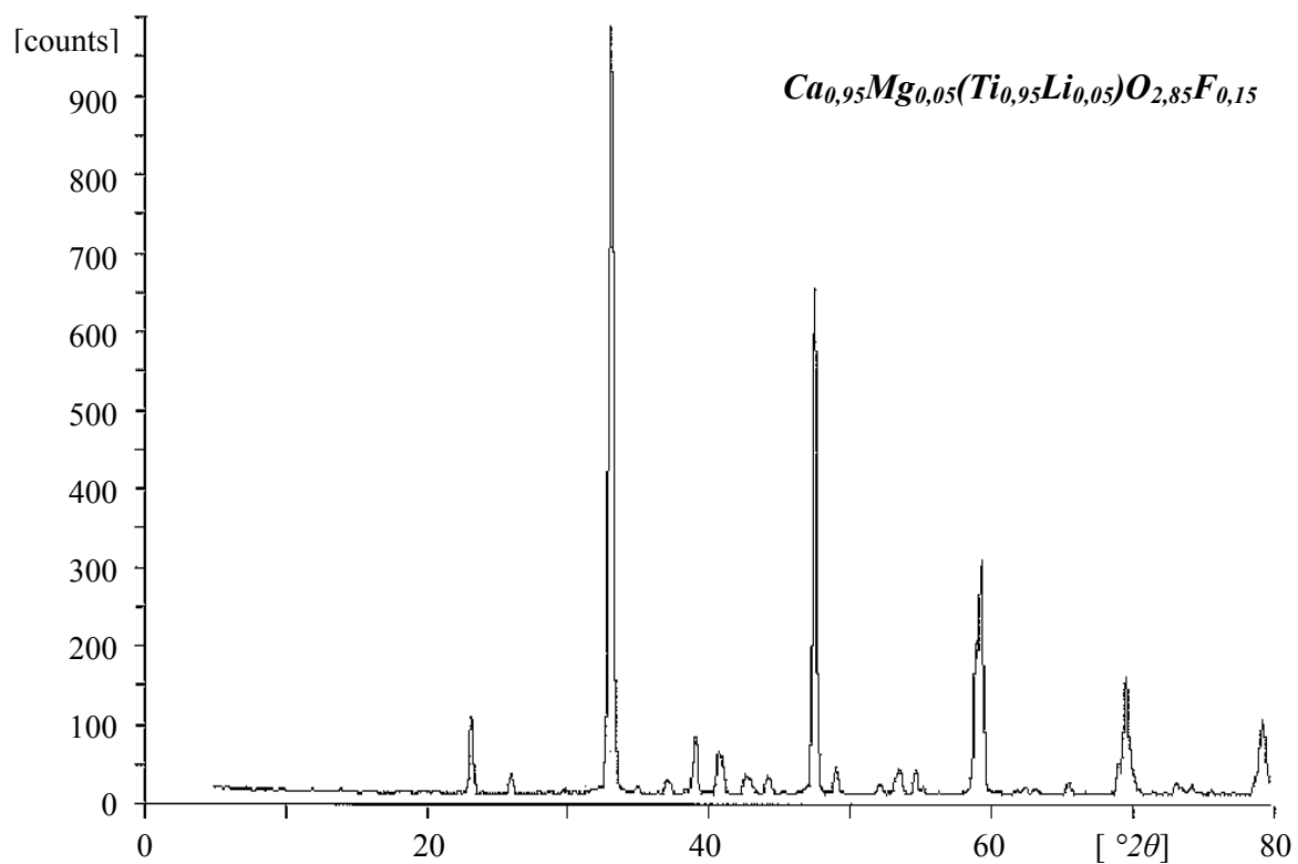
Figure 17: Spectres DRX à 300 K des phases oxyfluorées de composition
