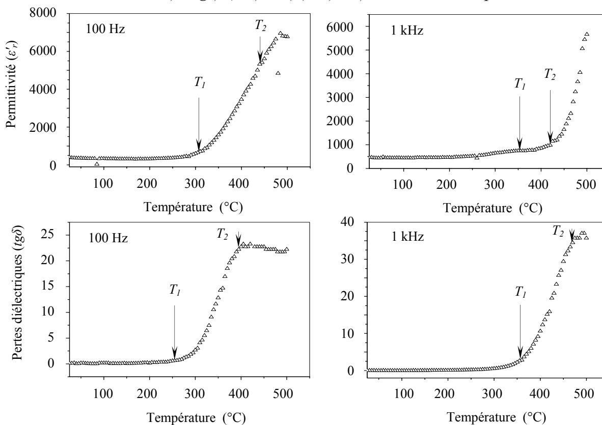
Figure 27: Variations de \epsilon'_r et tg\delta avec la température pour l'oxyfluorure
