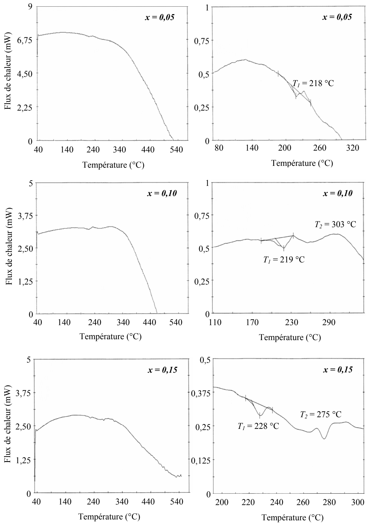
Figure 24: Courbes DSC des oxyfluorures Ca_{1-x}Mg_x(Ti_{1-x}Li_x)O_{3-3x}F_{3x} frittés à 900 °C pendant 2h
